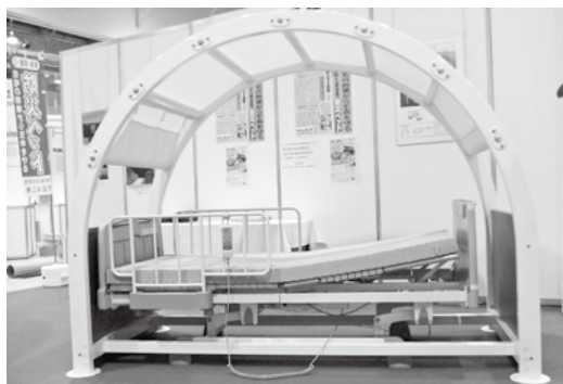
耐震ベッドの一例
