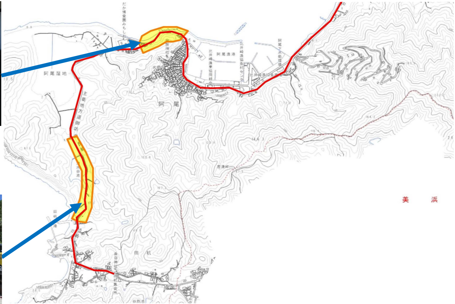
②-1 県道御坊由良線（田杭～阿尾）みちしお付近 幅員が狭く、線形も悪い。 強風により越波が発生する。 （改良工事を実施中）
